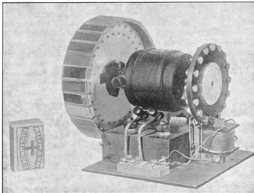
Het nieuwe Spiegelrad voor de Telefunken-Karolus Televisie-ontvangst, waarover wij in ons volgend nummer nadere bijzonderheden brengen
